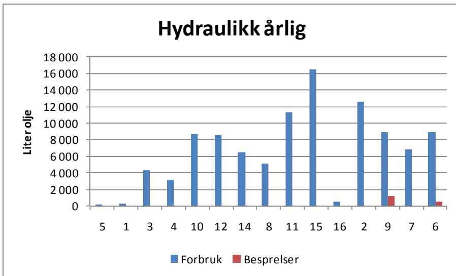
figur 73: Oljeforbruk og sparepotensial for hydraulikkanlegg i deltakerfartøyene
