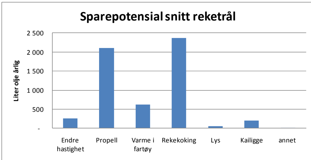
figur 53: Sparepotensial for fartøy med reketrål. Merk at det første og andre tiltaket innvirker på hverandre. Derfor blir summen av besparelsene beregnet ut fra det av tiltakene som gir mest reduksjon.
